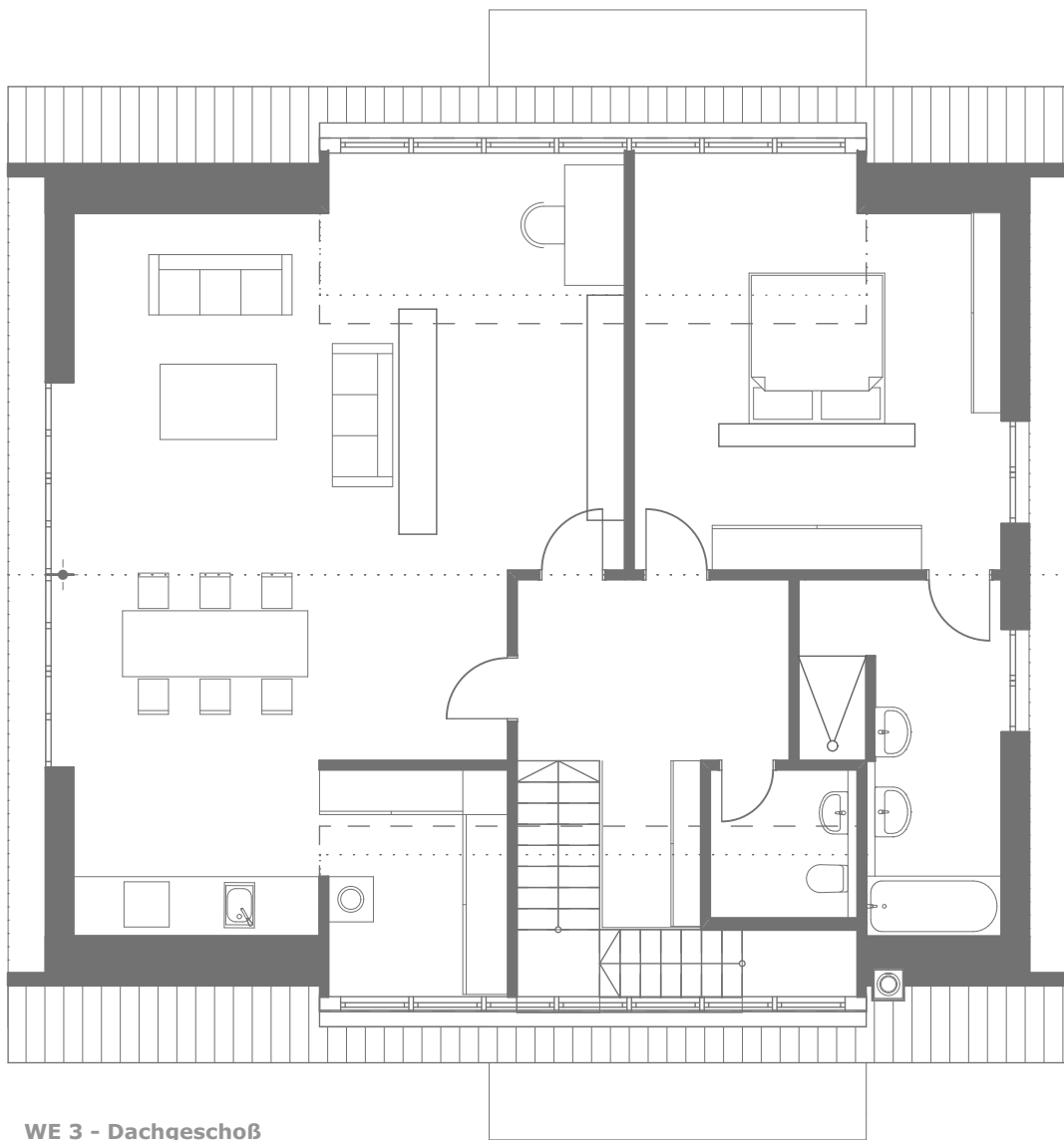
WE 3 - Dachgeschoß
