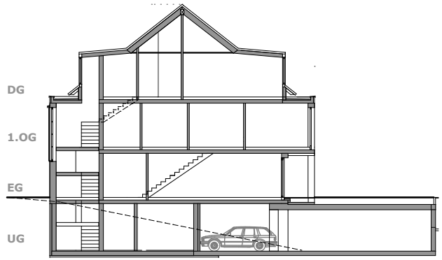
Querschnitt Treppenhaus
